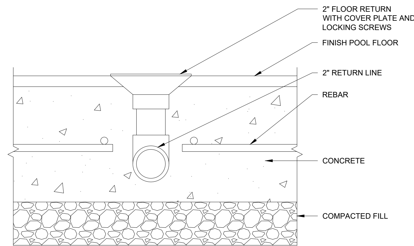
1 FLOOR RETURN SCALE: 3" = 1'-0"
