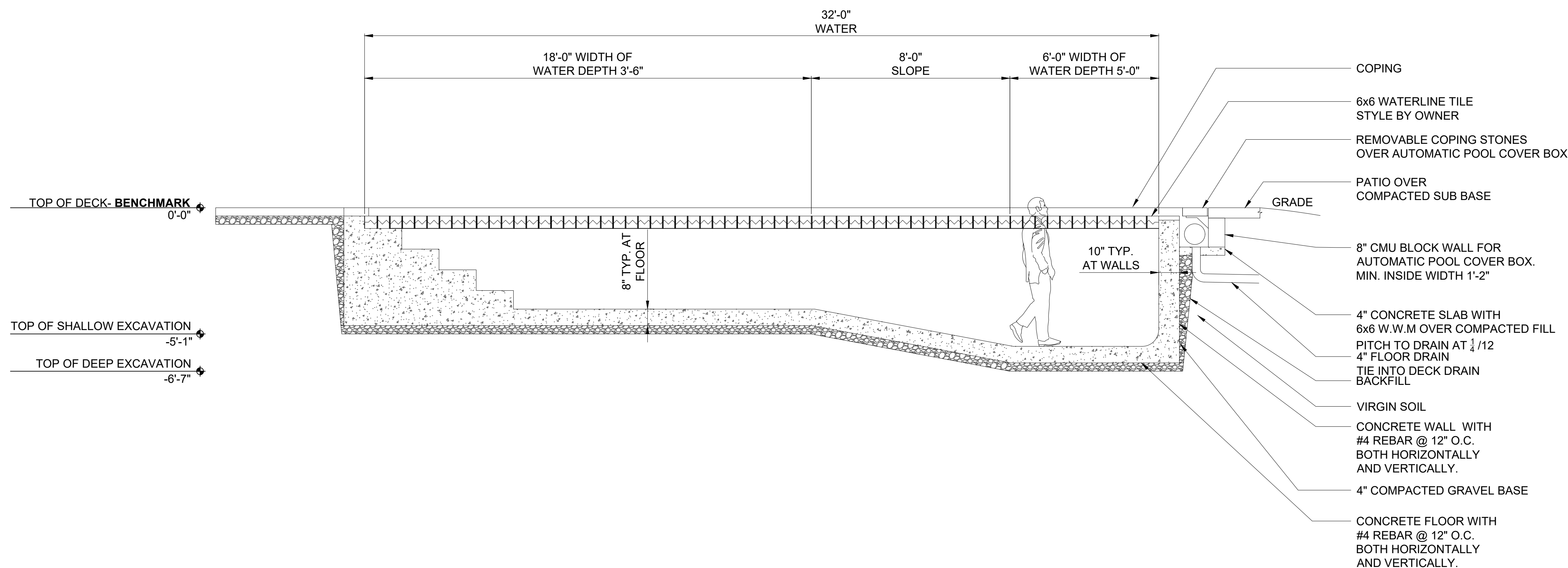
1 POOL SECTION SCALE: 3/8" = 1'-0"
